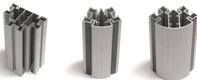
Montants pour traverses fixes avec départs en T, de 90° et 135°
